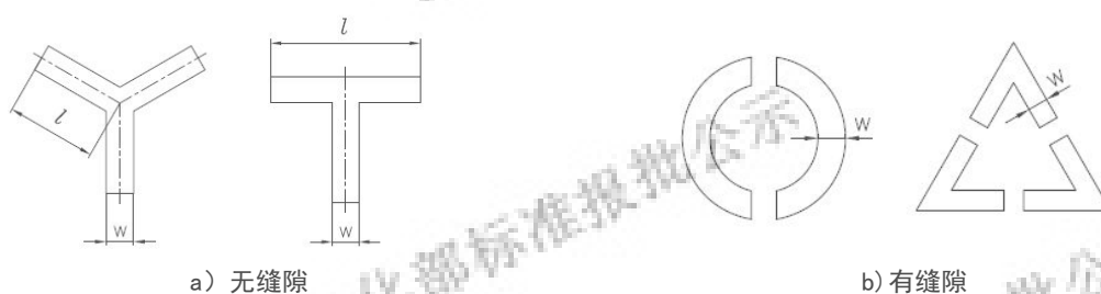
图4 异形微孔孔形
