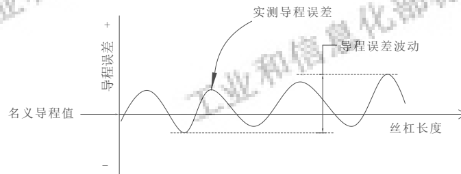
图 1 丝杠导程滚槽误差波动示意图
