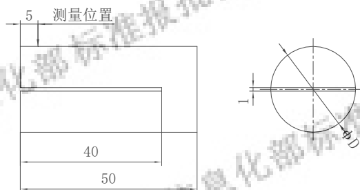
图5 切缝应力检测试样尺寸和检测位置示意图
