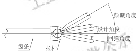
图7 齿条弯曲受力方向图
