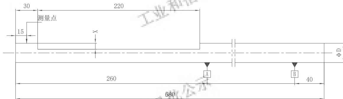
图 3 单齿应力检测尺寸和检测位置示意图
