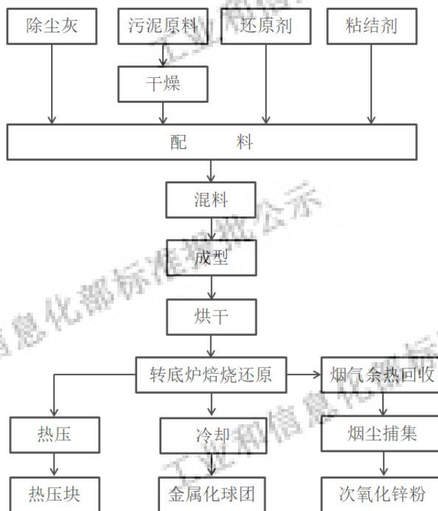
图1 典型转底炉处理冶金尘泥工艺流程
