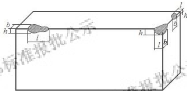
图2 缺棱掉角测量示意图
