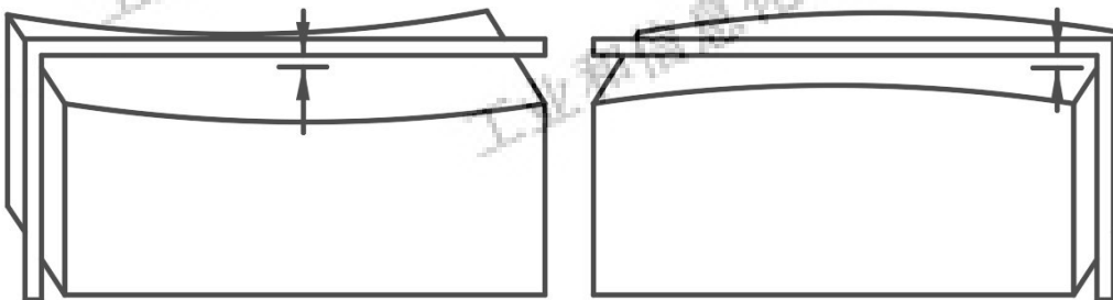
图3 平面弯曲测量示意图
