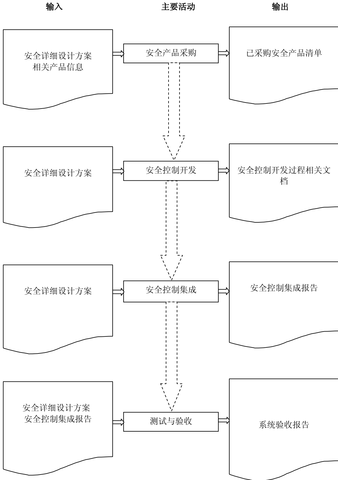
图 8-3 等级保护技术实施基本流程
